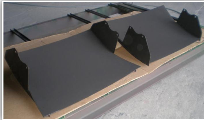
Cuillères de Goulotte rectifiées et revêtues au Téflon-PTFE
